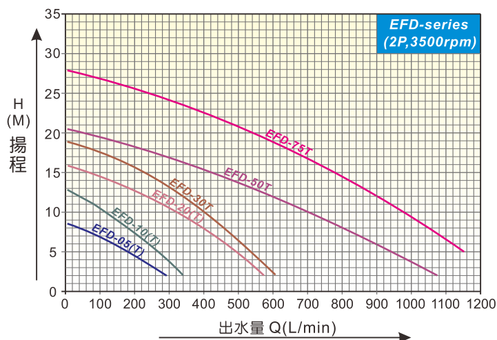
不阻塞泵葉 附SUS316攪拌棒
